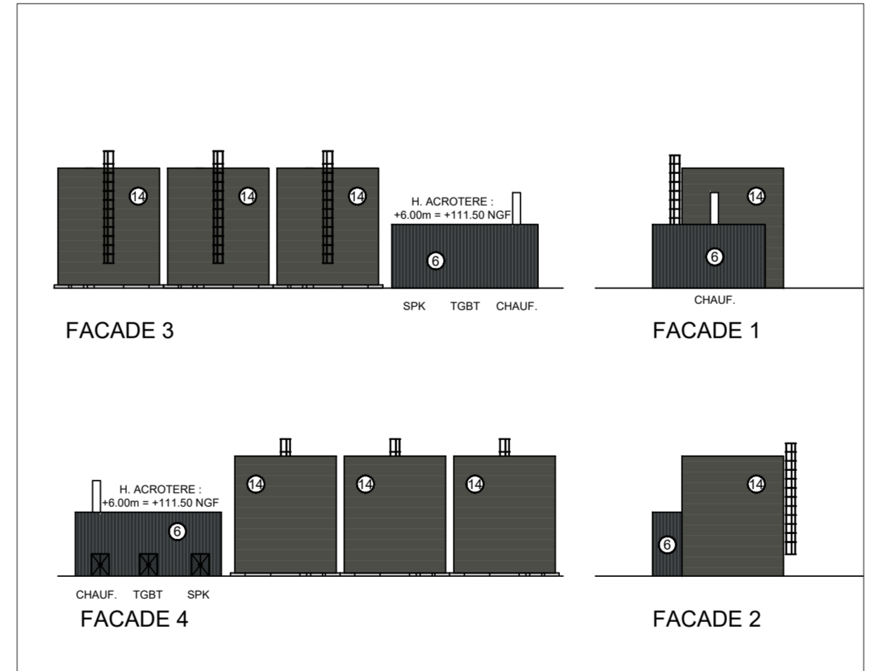
FACADES LOCAUX TECHNIQUES - Ech. : 1/500ème
