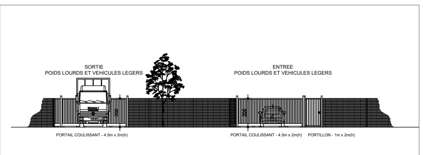
ACCES AU SITE n°1 - Ech. : 1/150ème
