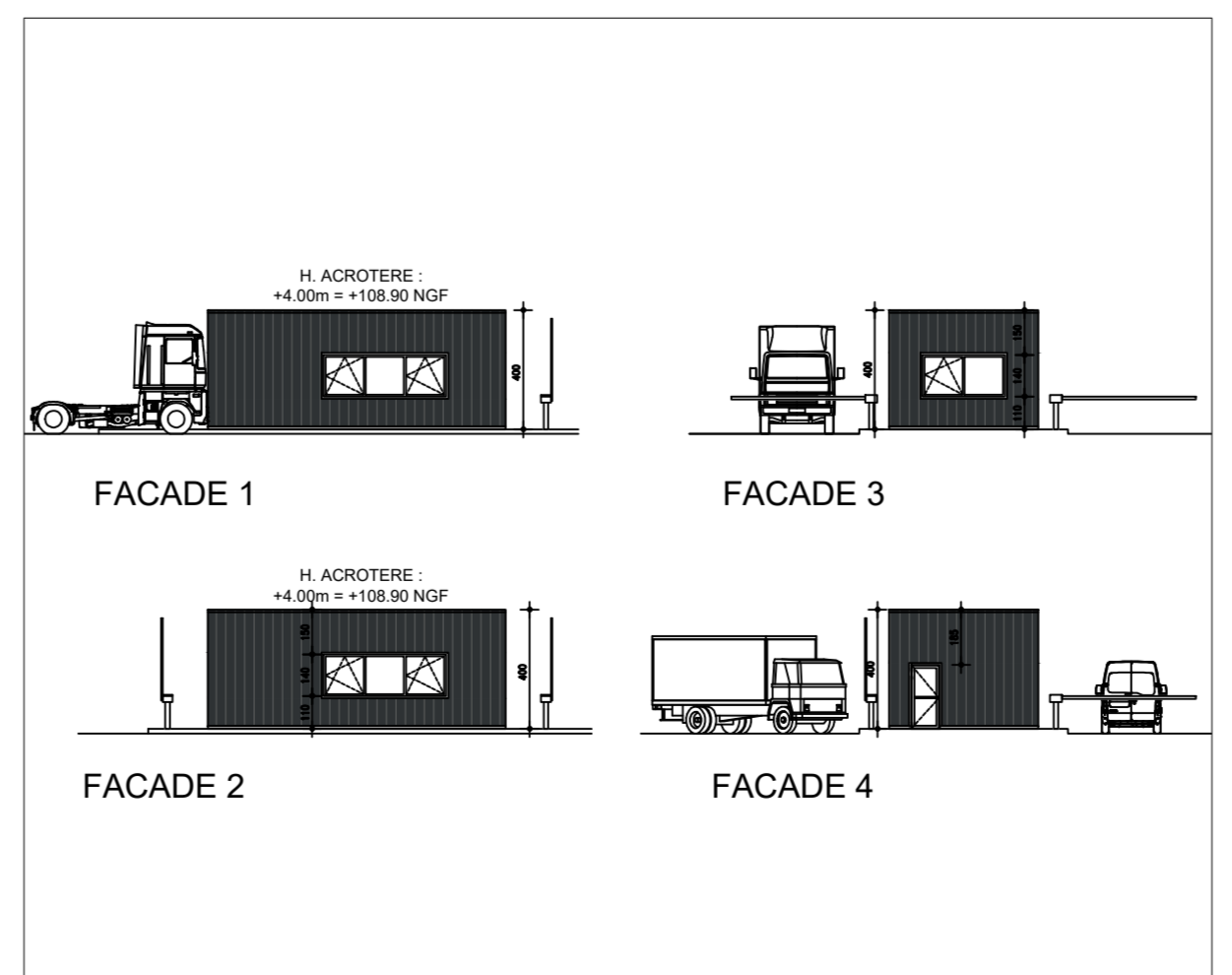
FACADES POSTE DE GARDE - Ech. : 1/250ème
